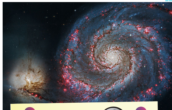
M51: Galaxias en interacción
